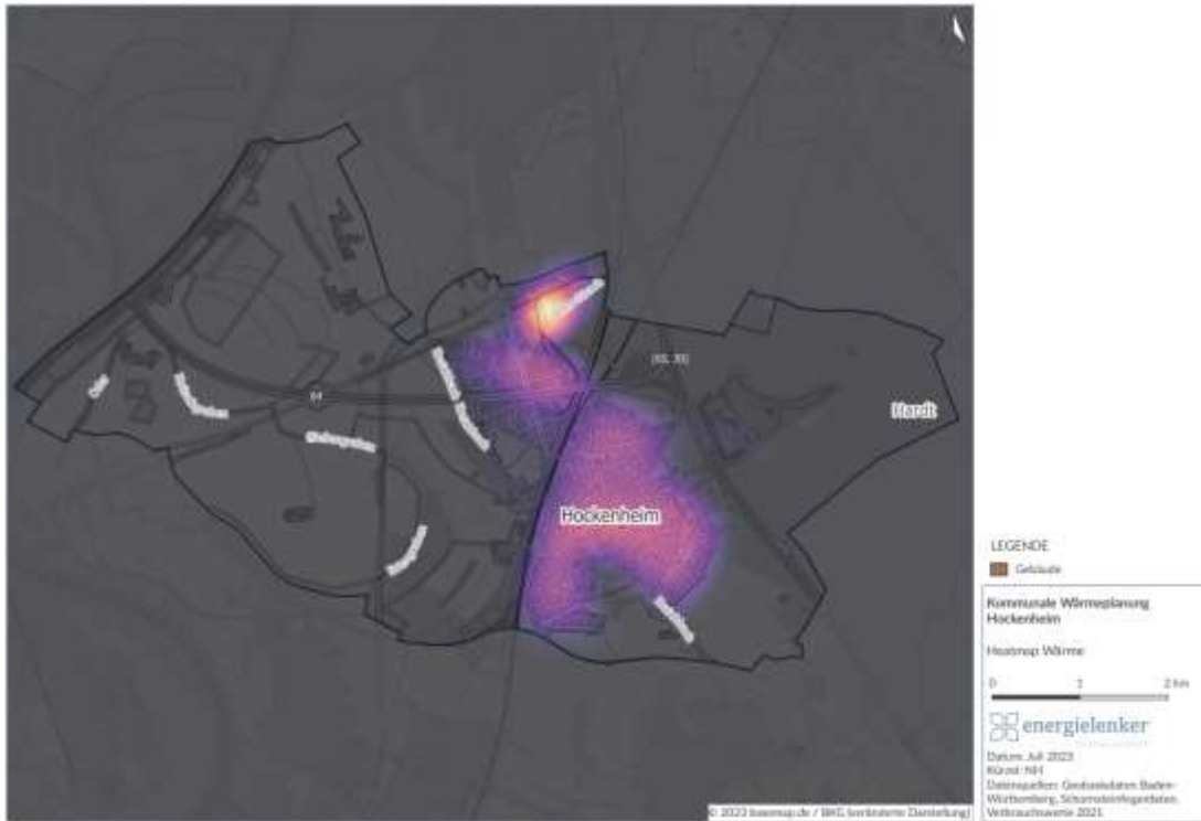
Abbildung 3-8: Heatmap des Wärmebedarfs der Stadt Hockenheim
