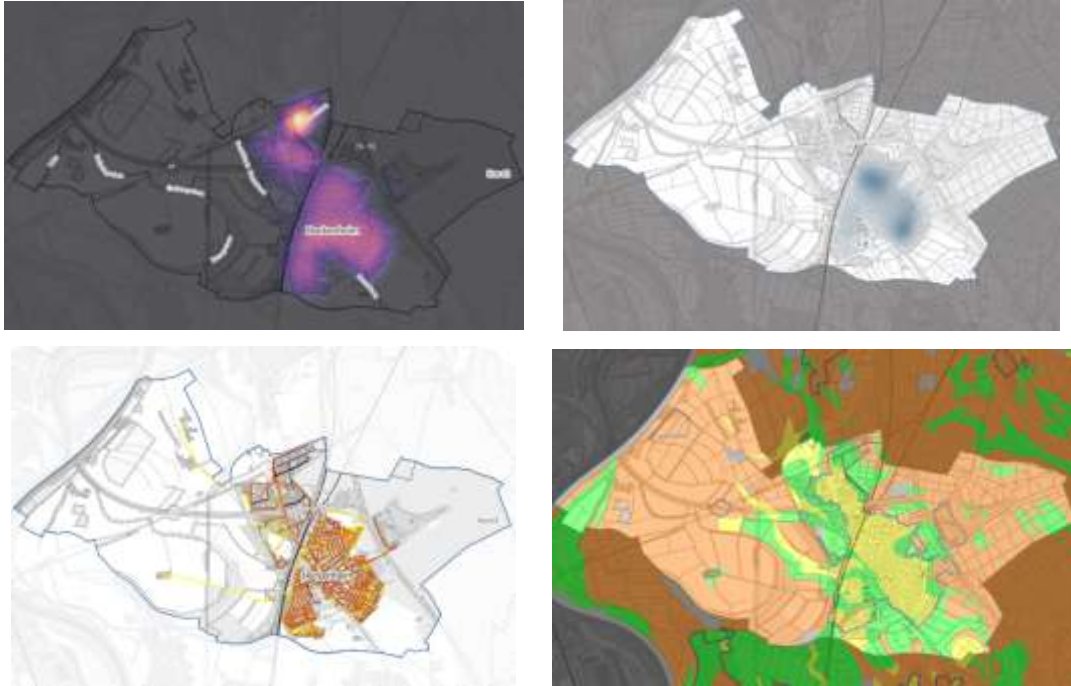
Abbildung 7-1: Kartenzusammenstellung: Heatmap - Wärmebedarf, Heatmap - Anzahl Ölheizungen, Wärmelinien-dichte, Erdwärmekollektorpotenzial (energielenker projects GmbH)
