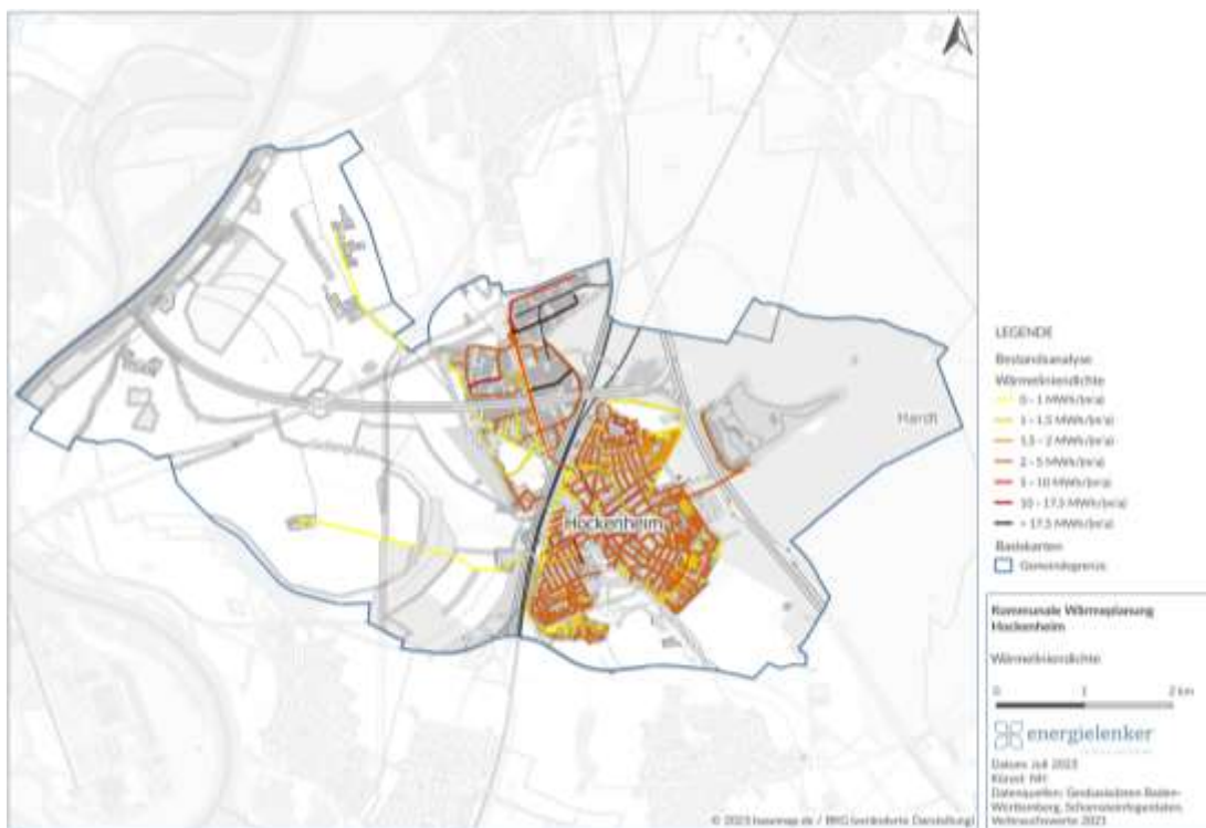
Abbildung 3-9: Wärmeliniendichten der Stadt Hockenheim
