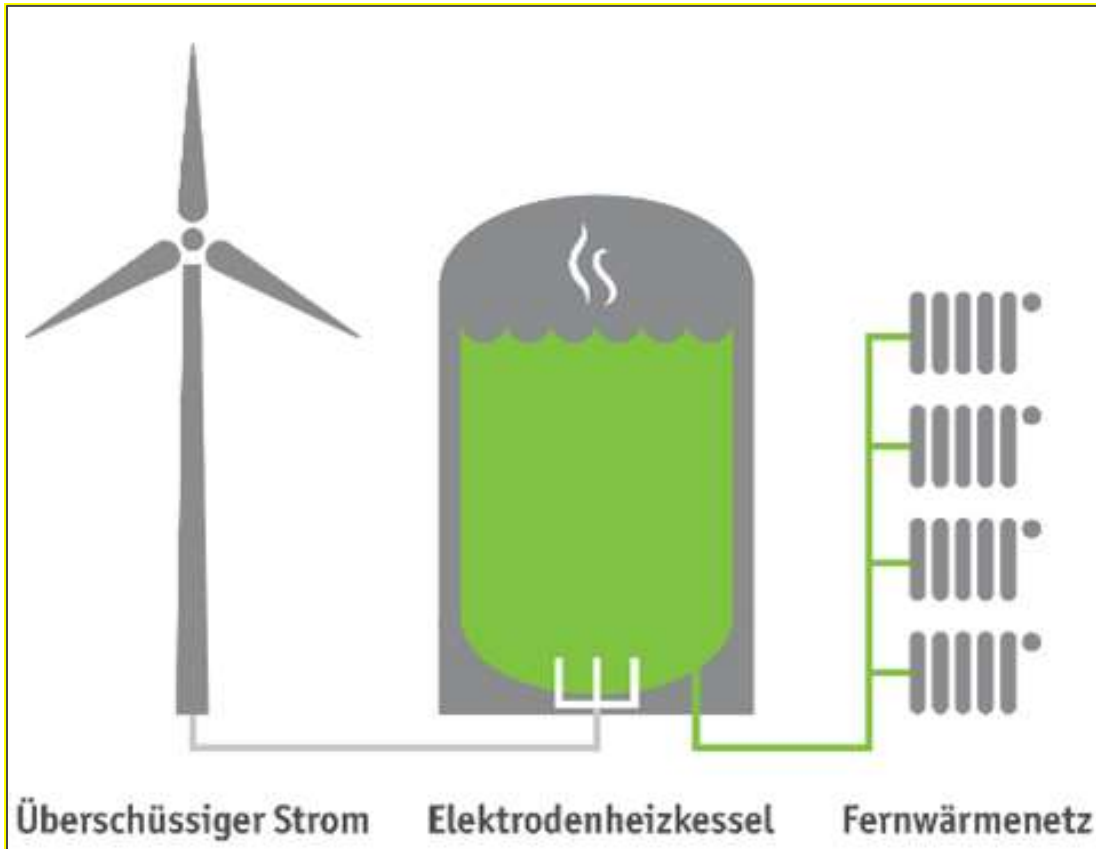
Abbildung 4-9: Funktionsweise Elektrodenheizkessel (Flensburg, kein Datum)
