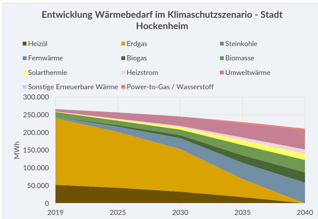
Abbildung 6-3: Entwicklung Wärmebedarf im Klimaschutzscenario (Quelle: energielenker projects GmbH)
